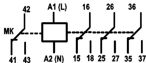
Рис 3. Схема включения реле. Контакты реле 41,42,43 устанавливаться опционально.
